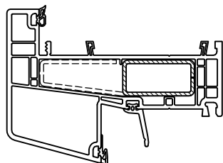
6802 bovendorpel
