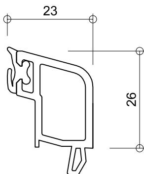
6140 glasdikte 39+40mm
