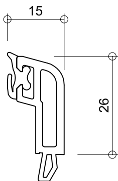
6148 glasdikte 47+48mm
