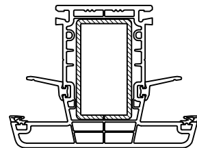
6054 tussenstijl
