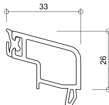
6130 glasdikte 29+30mm
