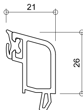
6142 glasdikte 41+42mm
