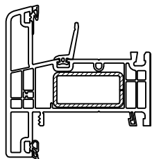
6070 onderdorpel
