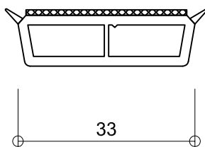
3195 glasroede 33mm
