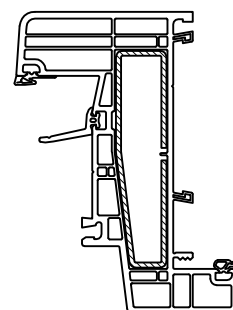
6808 buitendraaiend
