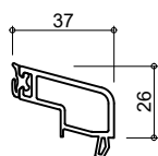
6126 glasdikte 25+26mm
