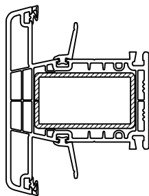
6054 tussendorpel
