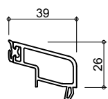
6124 glasdikte 23+24mm
