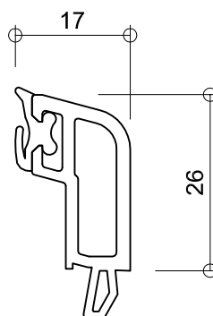
6146 glasdikte 45+46mm
