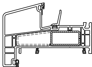
6802 onderdorpel
