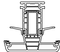
6050 tussenstijl
