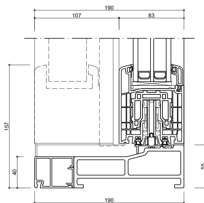
glasvezel versterkte HS-dorpel - hoogte 55mm - kleur zwartgrijs
