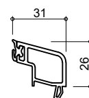
6132 glasdikte 31+32mm
