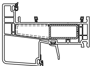
6804 bovendorpel
