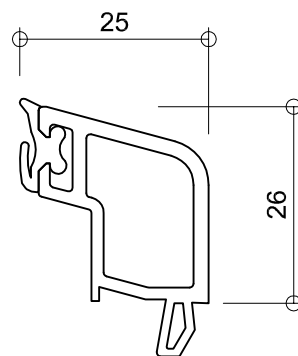
6138 glasdikte 37+38mm
