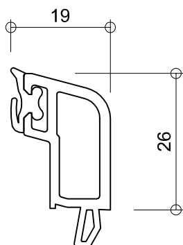
6144 glasdikte 43+44mm
