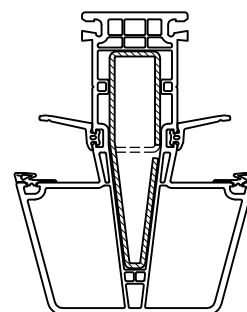
6816 tussenstijl
