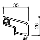
6128 glasdikte 27+28mm
