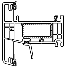
6070 bovendorpel
