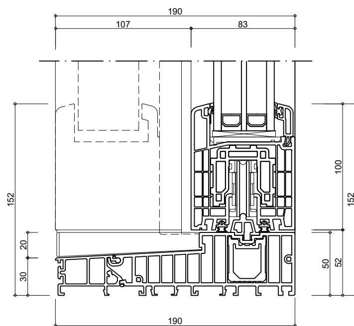
Siegenia Ecopass HS-dorpel - hoogte 50mm - kleur grijs
