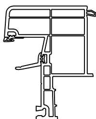
6844 adapter t.b.v. buitendraaiend
