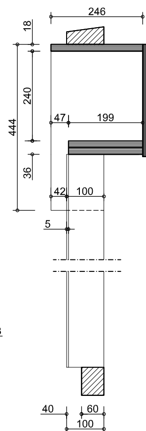
doorsnede
