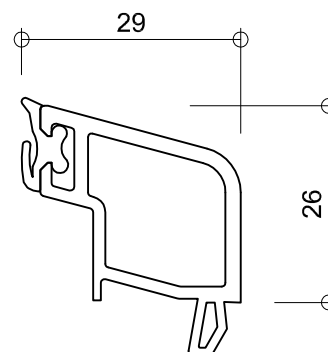
6134 glasdikte 33+34mm
