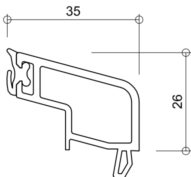
6128 glasdikte 27+28mm
