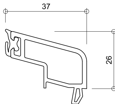
6126 glasdikte 25+26mm
