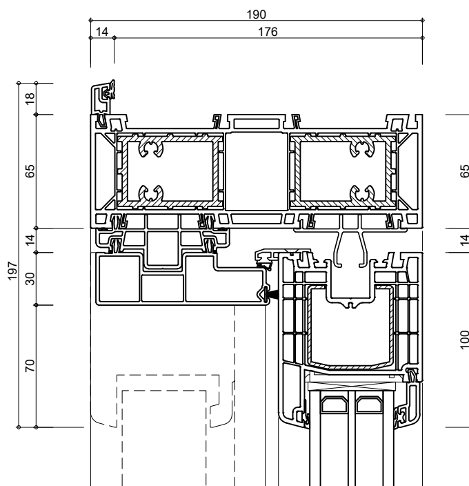
schuivend deel Standaard uitvoering
