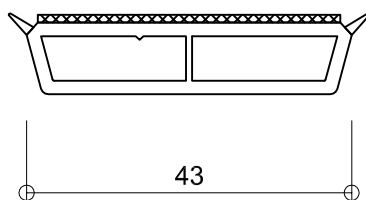
3198 glasroede 43mm
