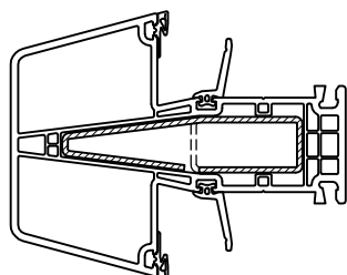
6816 tussendorpel
