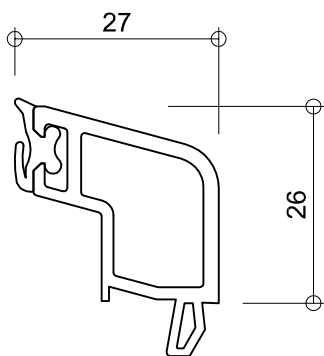
6136 glasdikte 35+36mm
