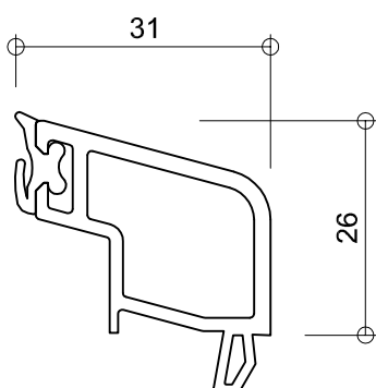
6132 glasdikte 31+32mm
