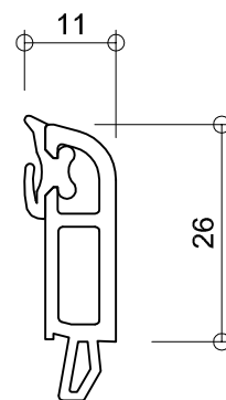
6152 glasdikte 51+52mm
