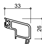
6130 glasdikte 29+30mm
